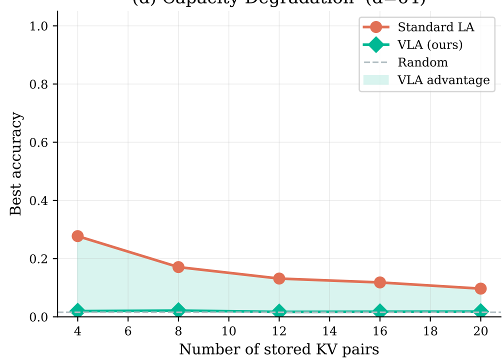
(d) Capacity Degradation ( d=64 )
