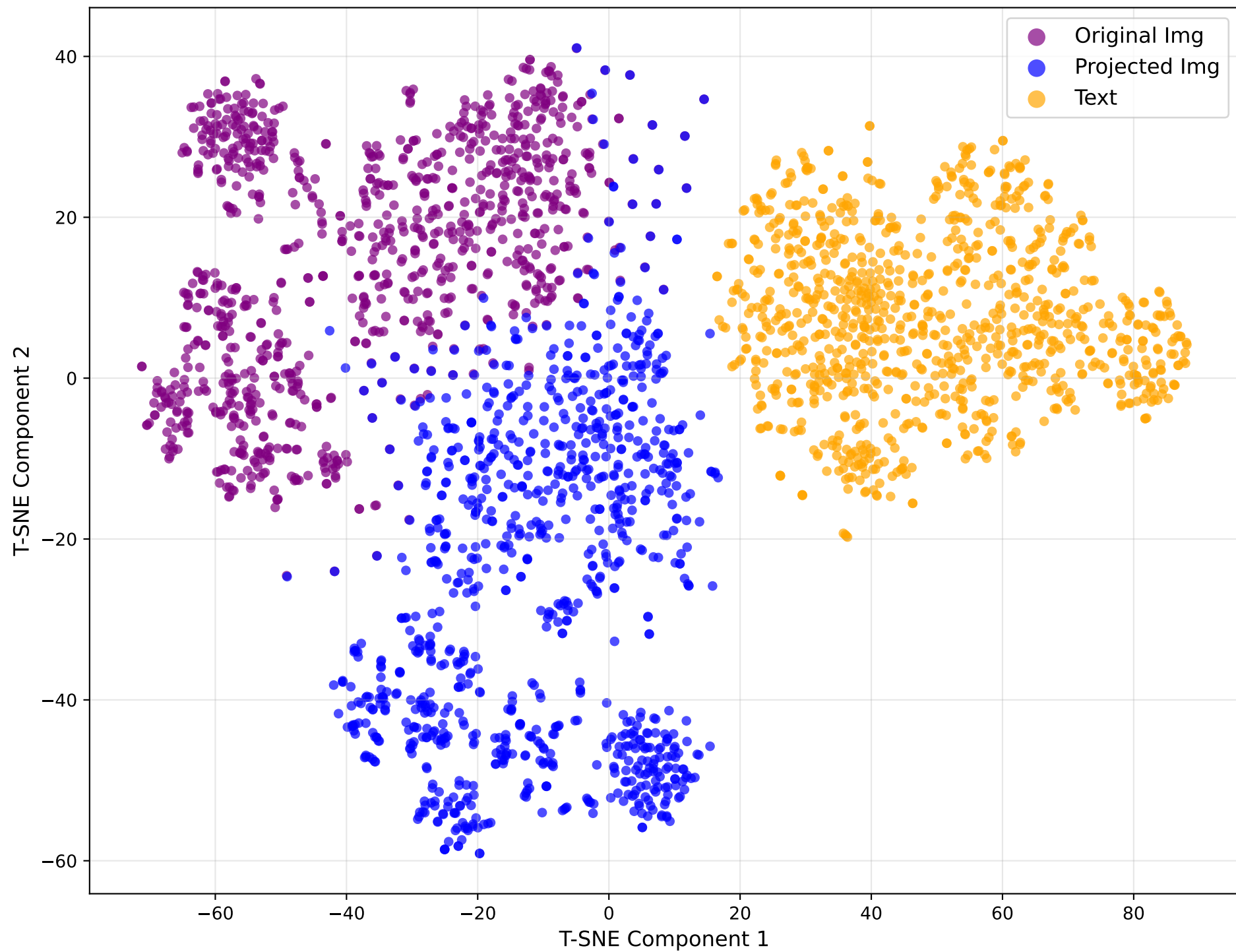
T-SNE
