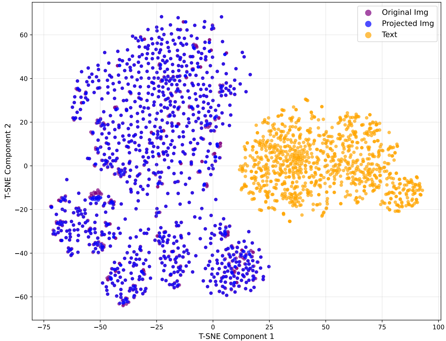
T-SNE
