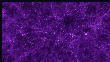
Cosmic web
