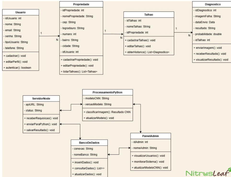
Figura 17: Diagrama de Classe
