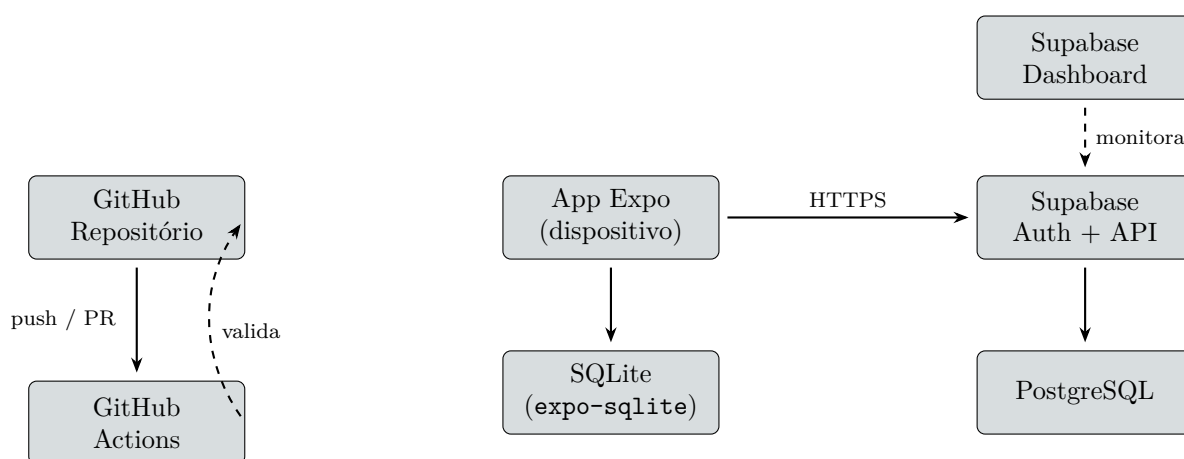
Figura 22: Arquitetura de deployment e monitoramento
