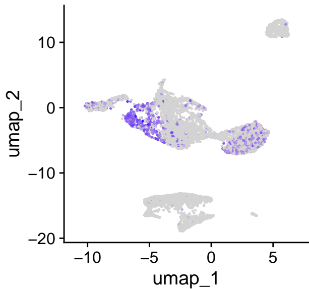
CD4
