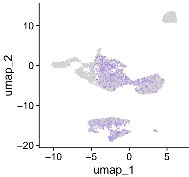
CD4
