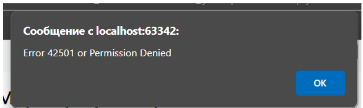
Рисунок 4 – Вывод сообщения
