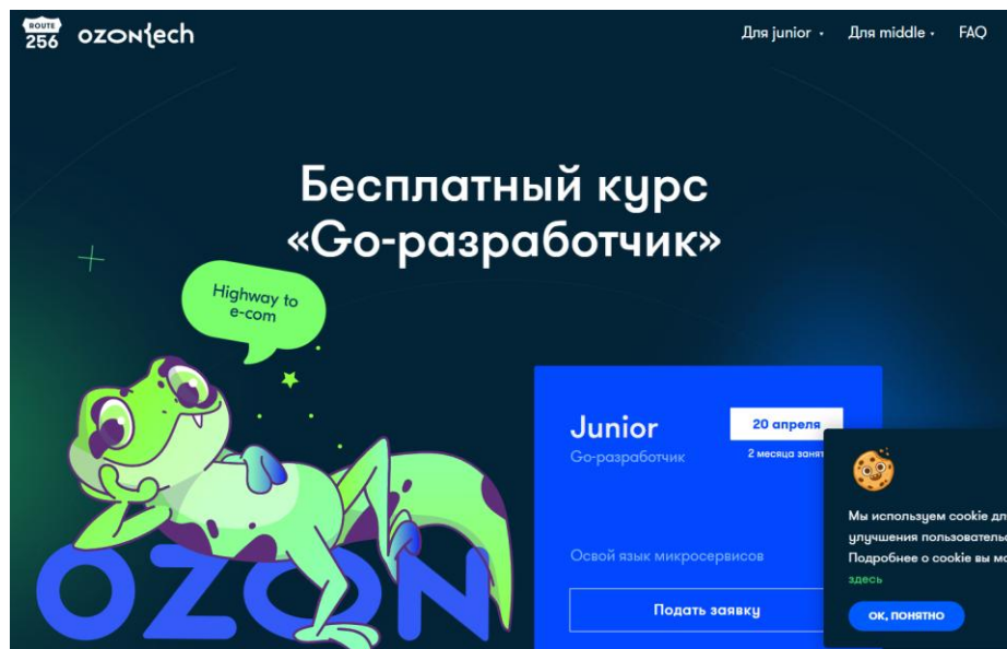
Рисунок 3 – Открытие страницы
