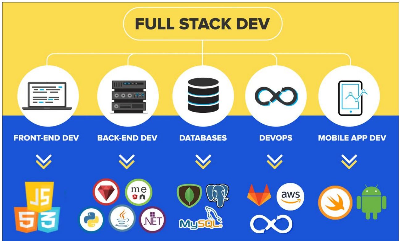
Рисунок 1 - Карта изображений
