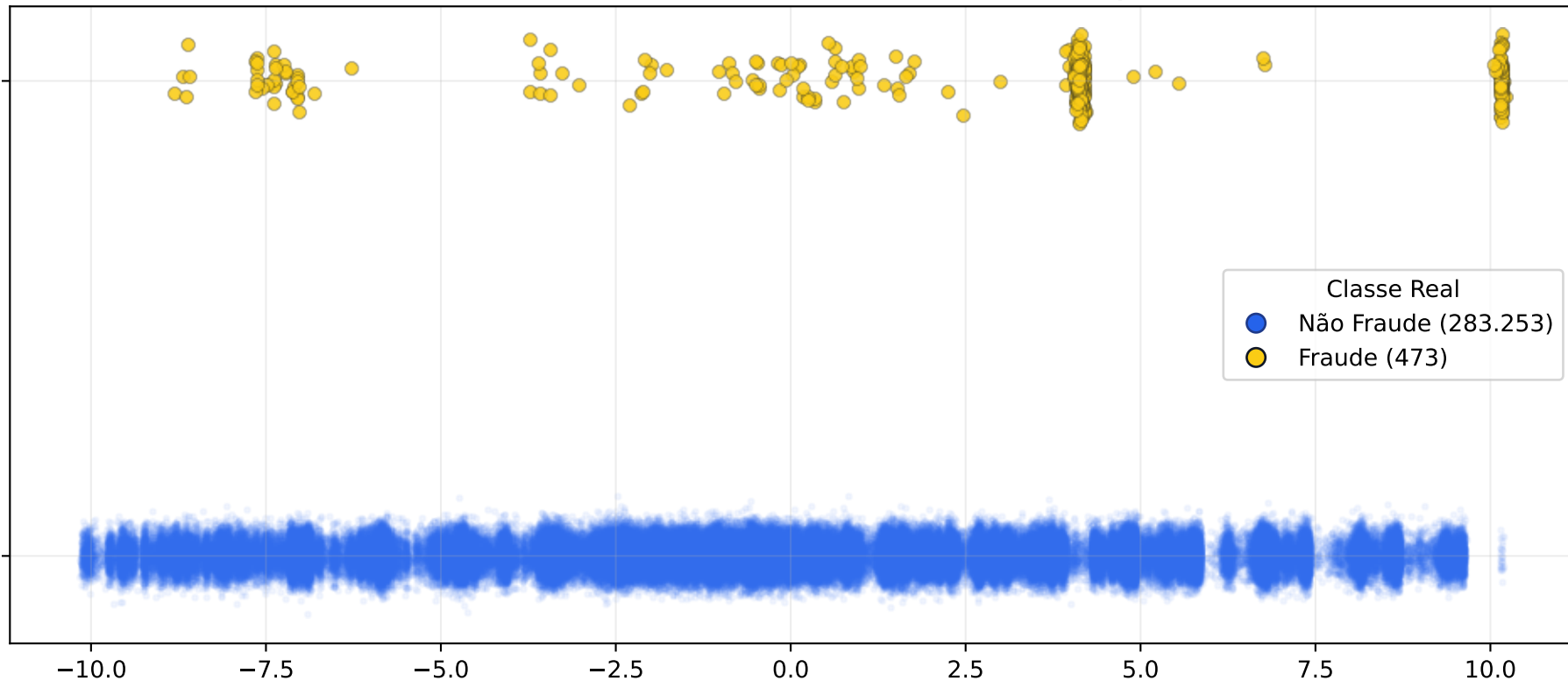
Representação 1D com 100% dos Dados - t-SNE 1D | Perplexity = 24
