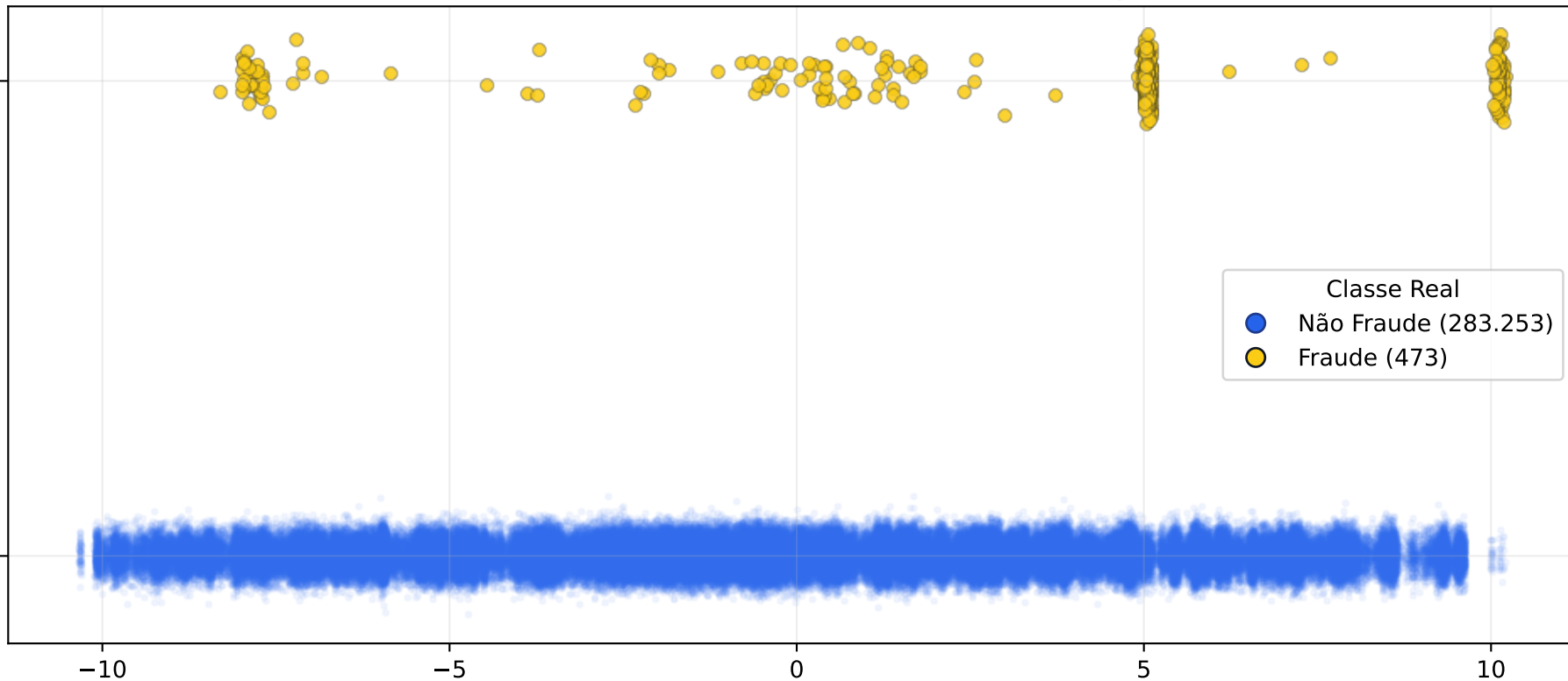
Representação 1D com 100% dos Dados - t-SNE 1D | Perplexity = 10
