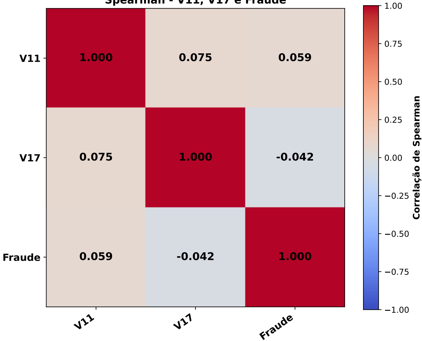
Spearman - V11, V17 e Fraude
