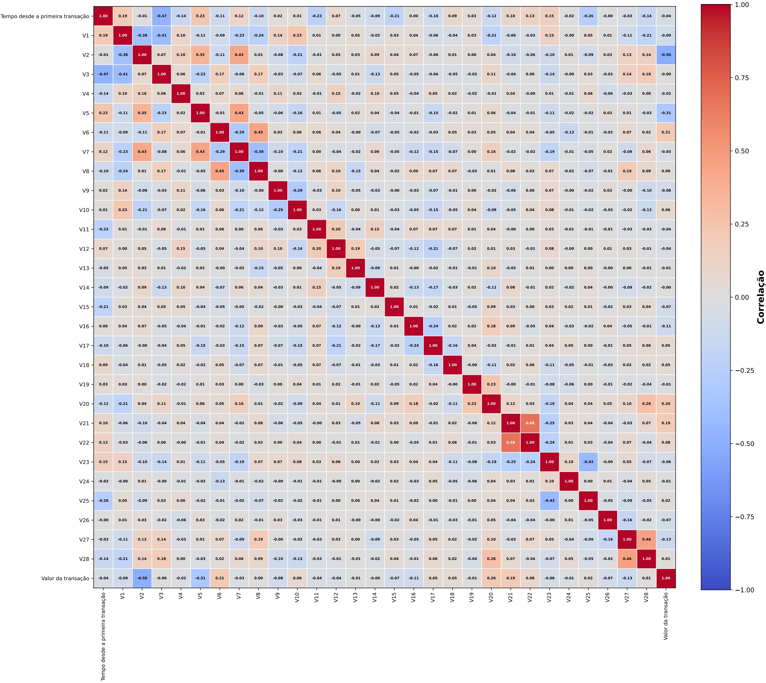
Matriz de Correlação de Spearman
