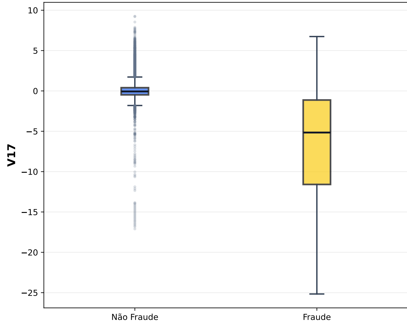
Boxplot - V17
