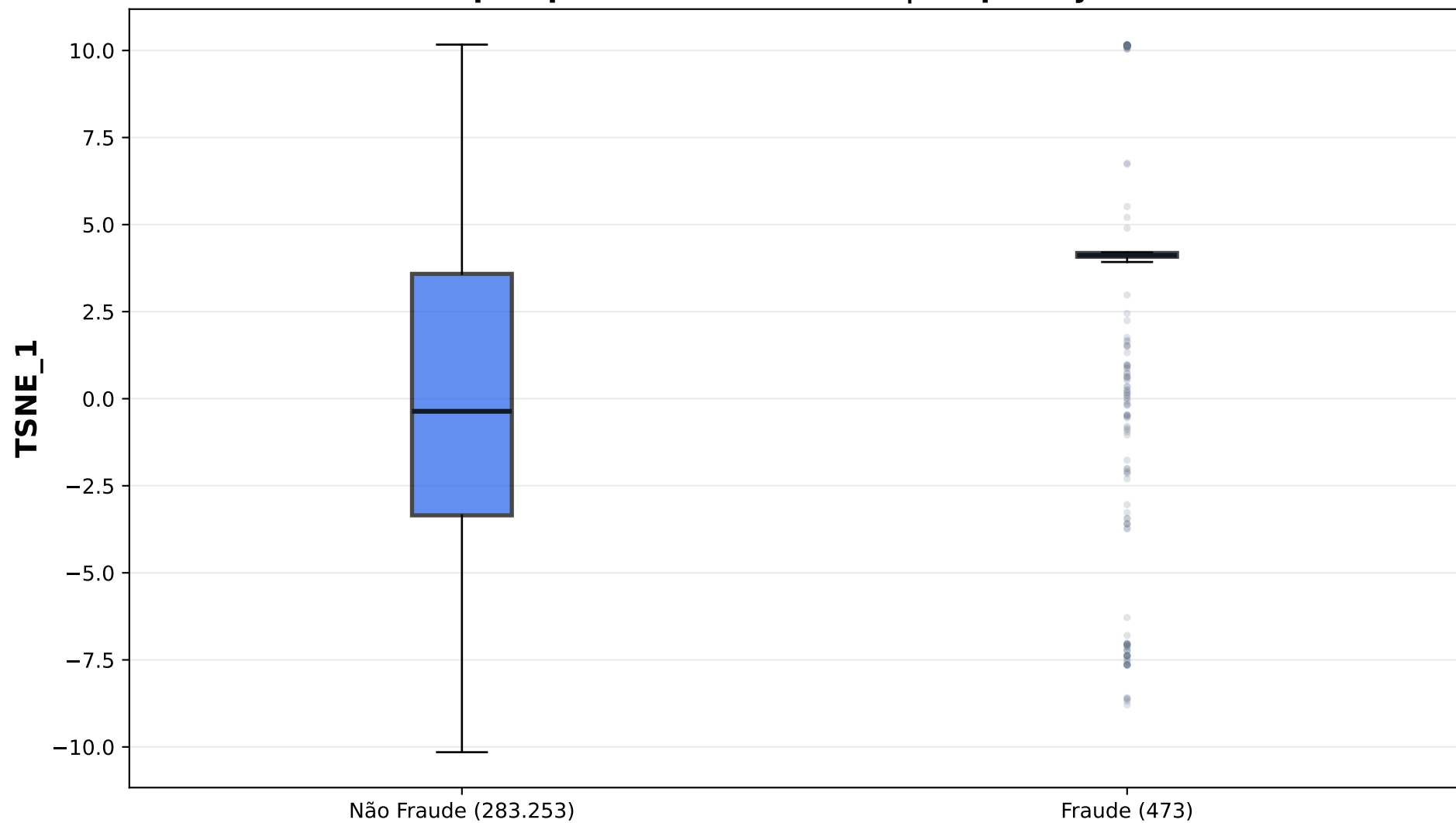
Boxplot por Classe - t-SNE 1D | Perplexity = 24
