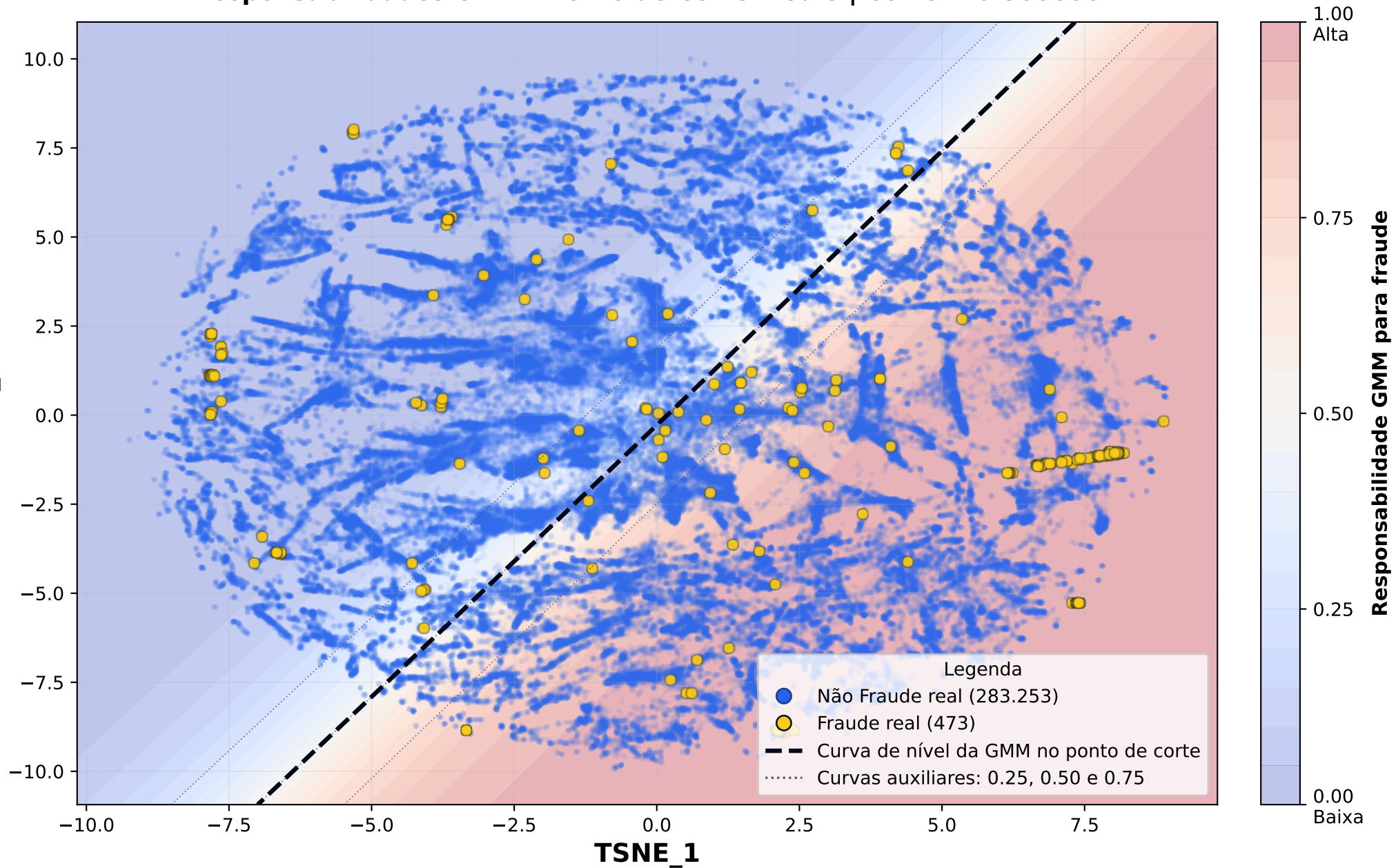
Responsabilidades GMM - Ponto de Corte Médio | Corte = 0.500000
