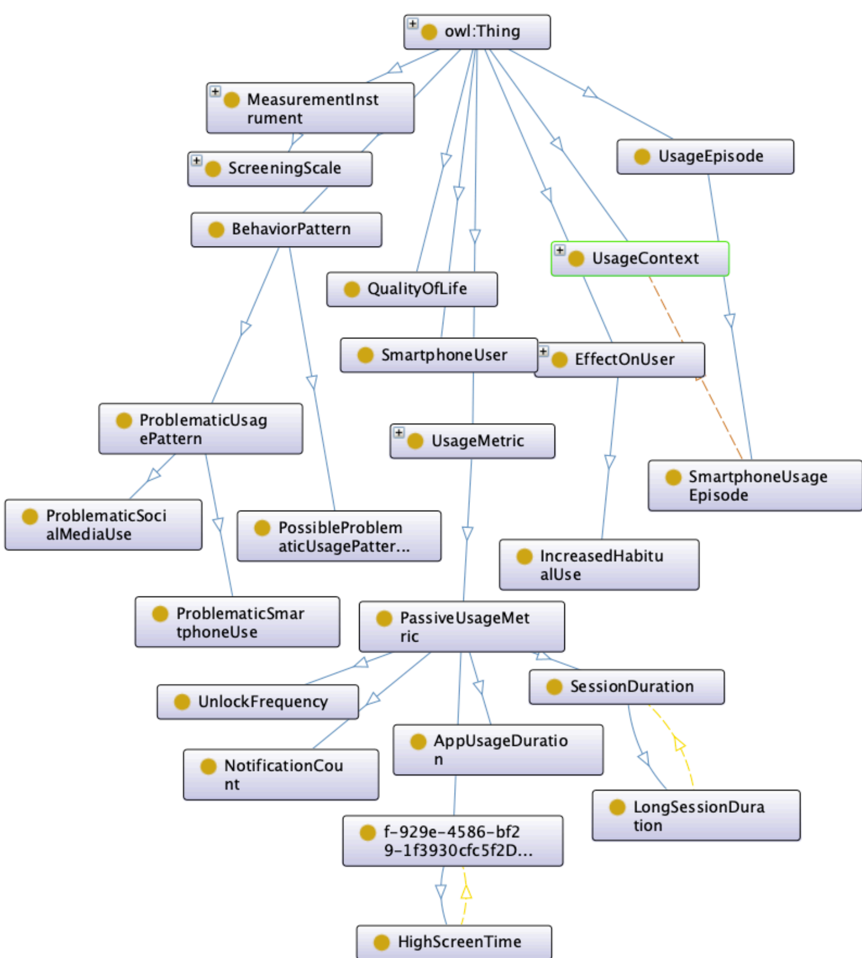
Figura 2 - Modelagem ontológica (Grafo Simplificado)
