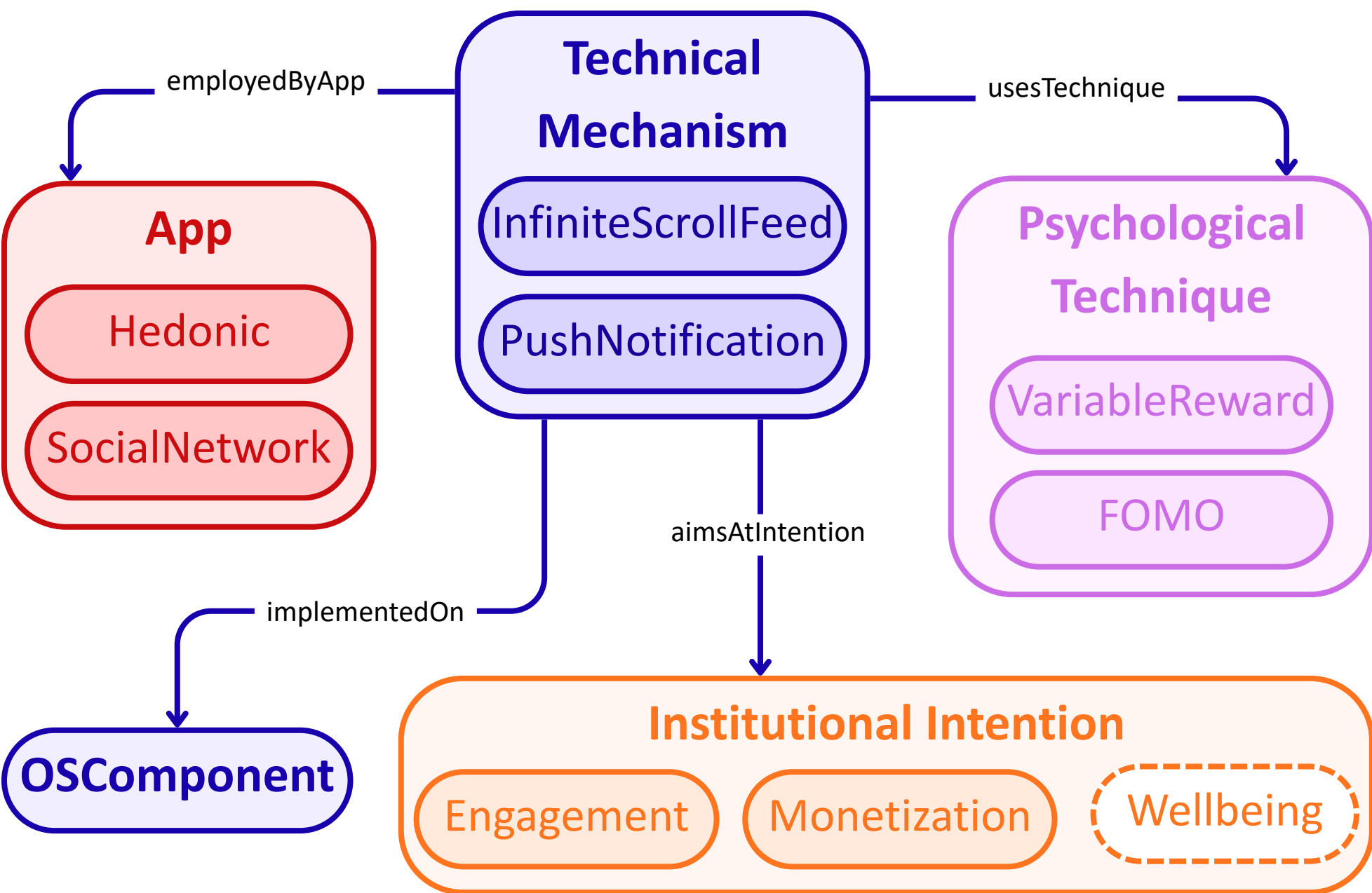
Figura 1 - Diagrama simplificado do ecossistema de retenção em smartphones
