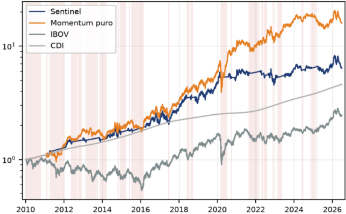
Curvas de patrimônio 2010-2026 (base 1,0; escala log; faixas = BEAR)
