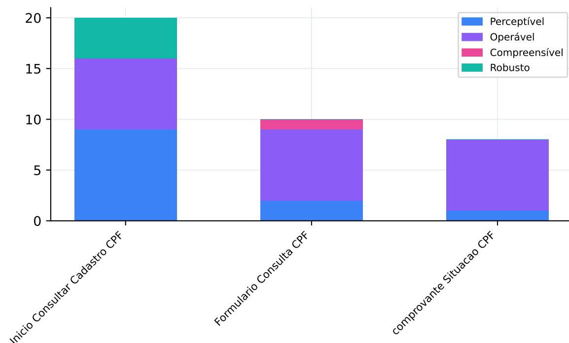
Dimensões POUR
