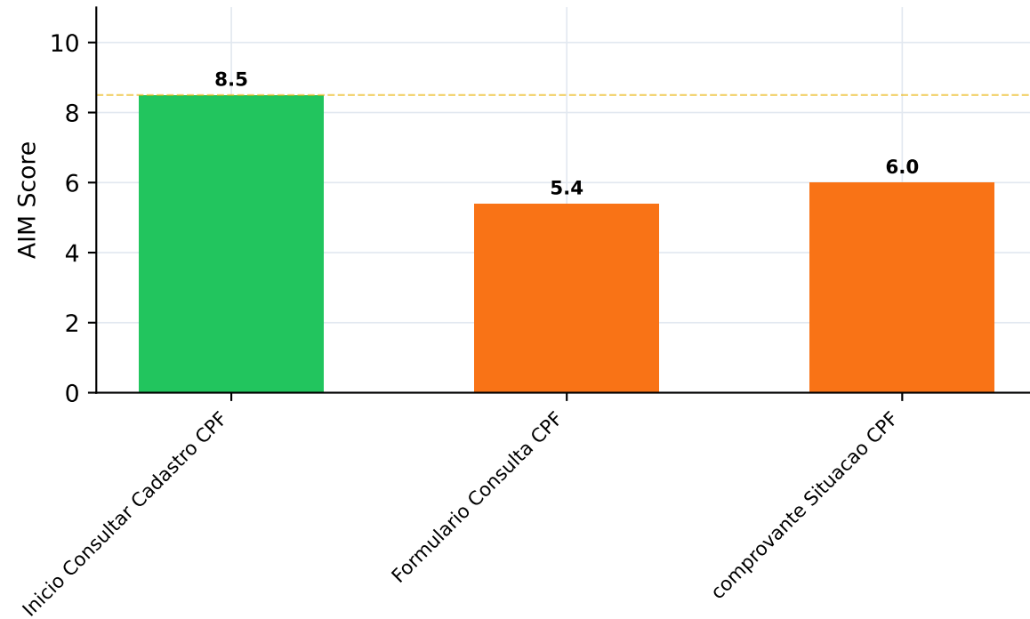
Pontuação AIM
