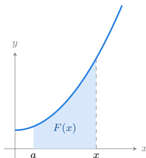
Figura 45.1.: A função área F(x) = \int_a^x f(t) dt ; o TFC diz que F'(x) = f(x) .
