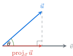
Figura 63.1.: O ângulo \theta entre \vec{u} e \vec{v} e a projeção de \vec{u} sobre \vec{v} .
