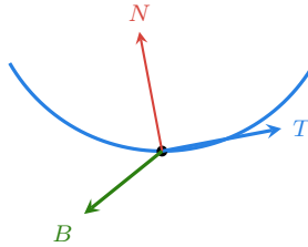
Figura 93.1.: O triedro de Frenet \{T, N, B\} : o referencial ortonormal que acompanha a curva.
