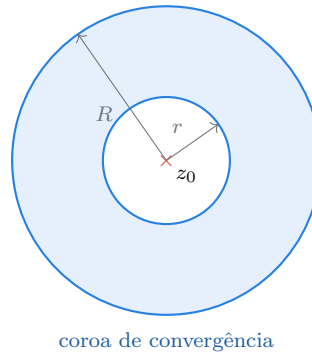
Figura 130.1.: A coroa r < |z - z_0| < R onde a série de Laurent converge.
