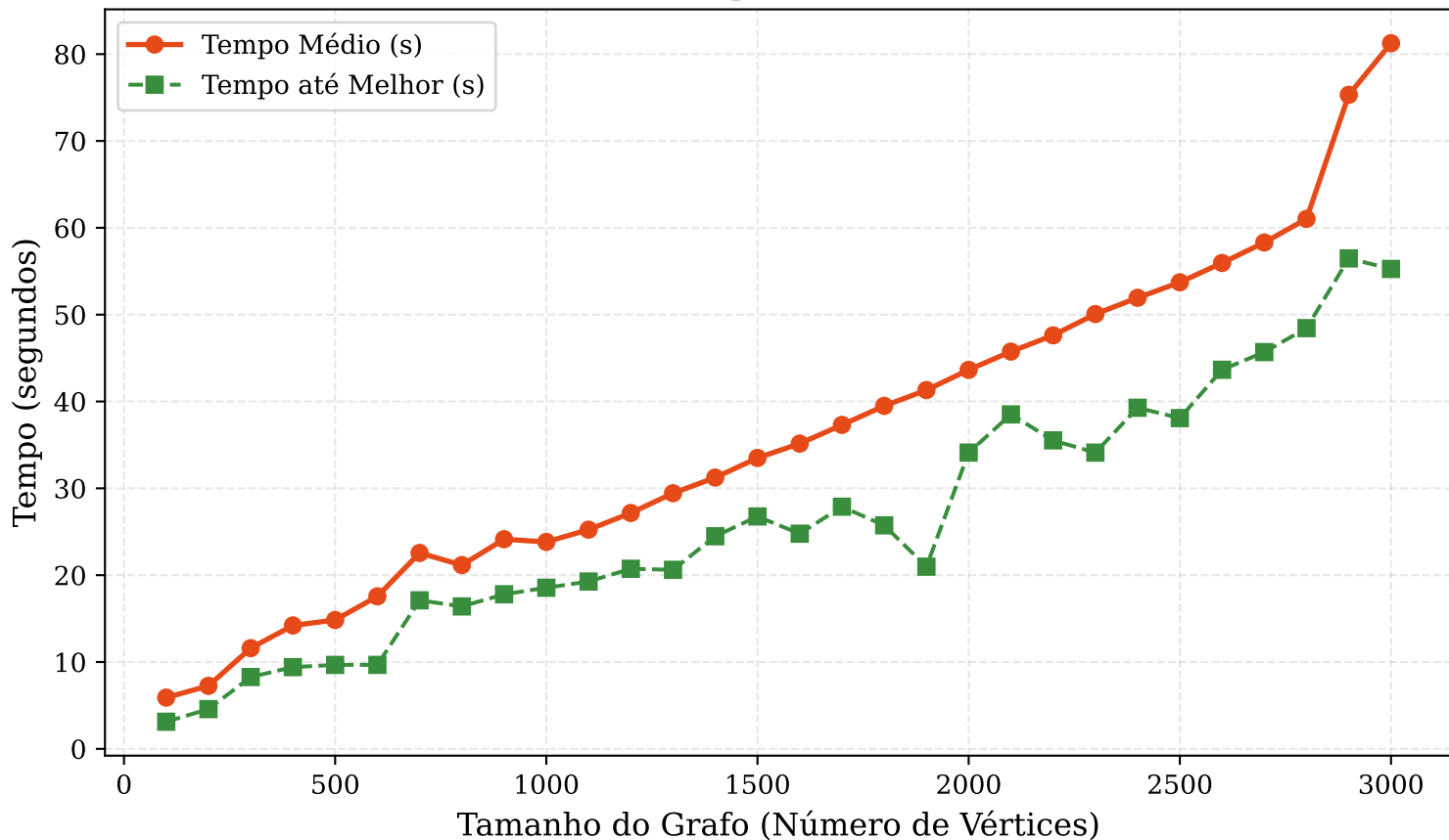
Escalabilidade de Tempo vs. Tamanho da Instância
