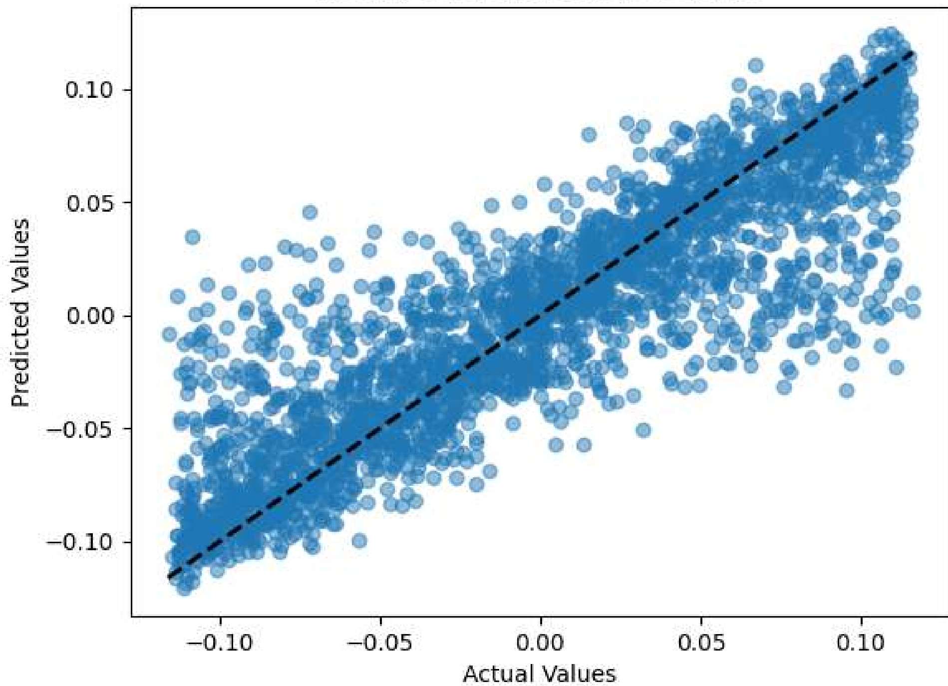
Actual vs Predicted for Output 1
