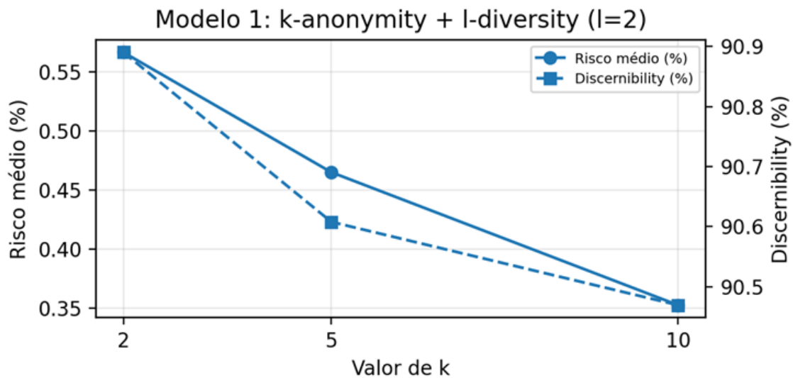
Figura 1 - Efeito do aumento de k no risco médio e na utilidade.
