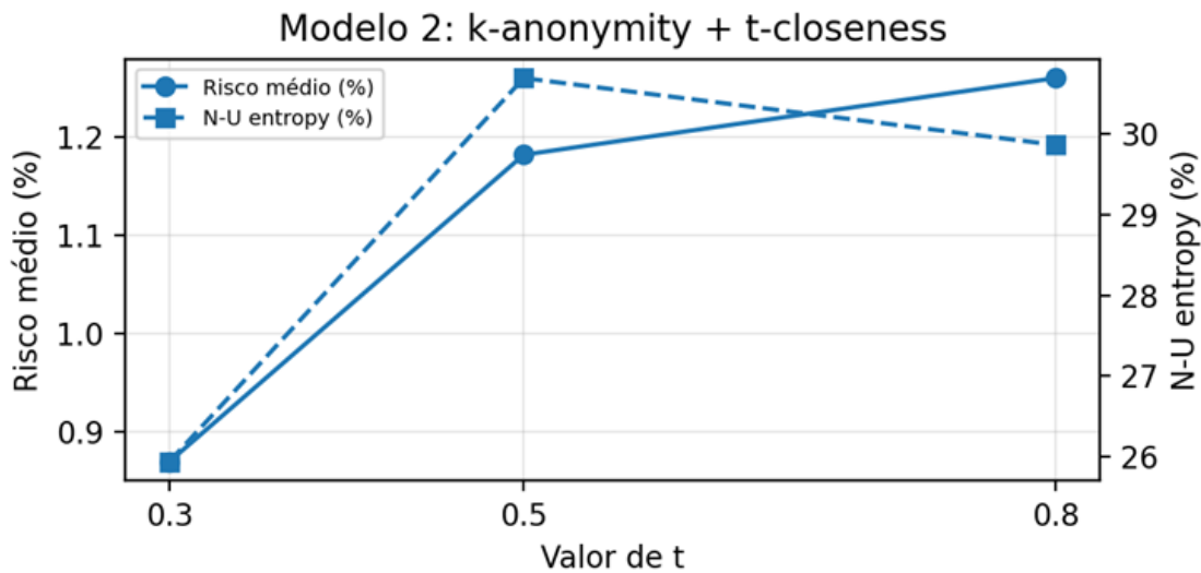
Figura 2 - Efeito da variação de t no risco médio e na N-U entropy.
