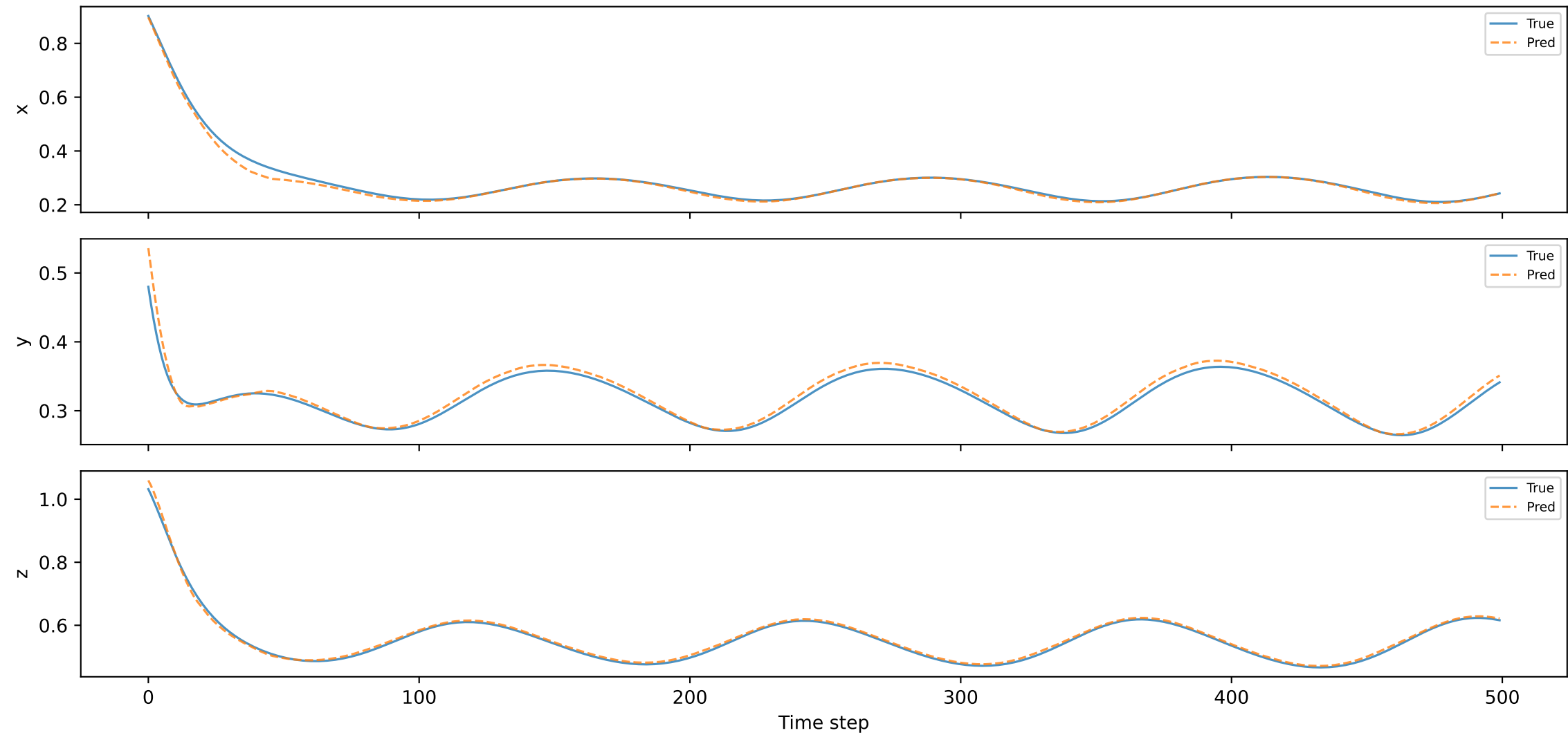
MAML - MS
