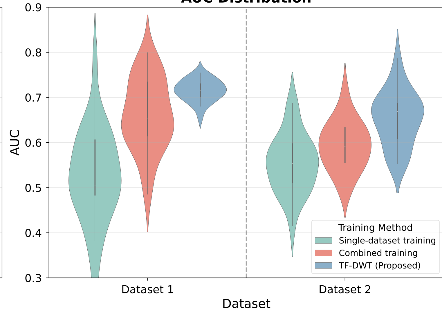
AUC Distribution
