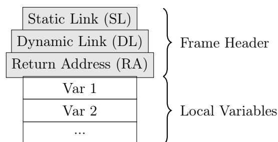
Gambar 2.2: Ilustrasi stack frame dengan static link, dynamic link, dan return address
