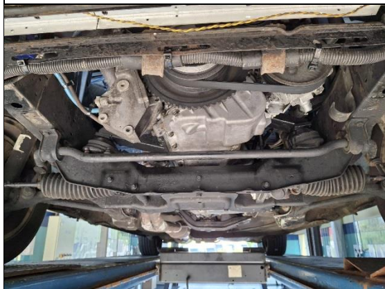
Fot. 5. Miejsce montażu jednostki napędowej
