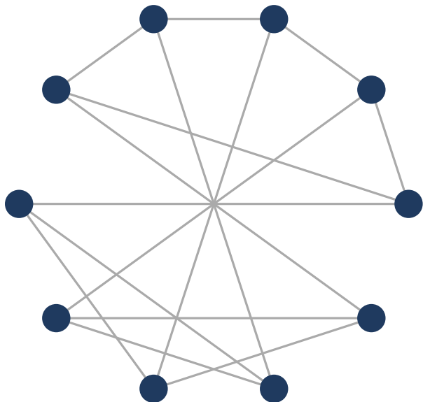
Petersen — (3,5)
