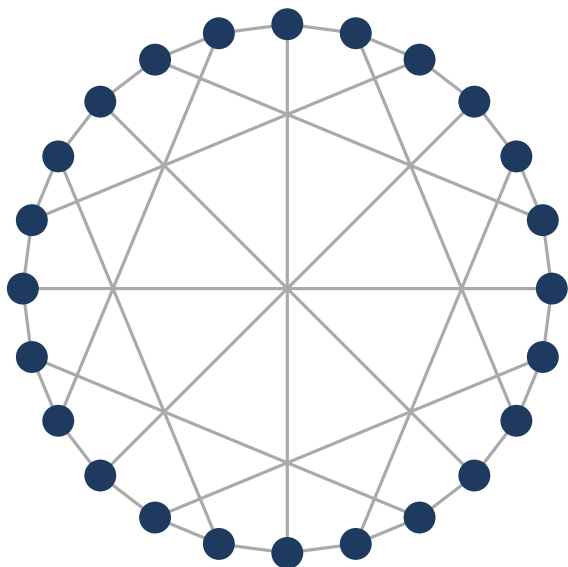
McGee — (3,7)
