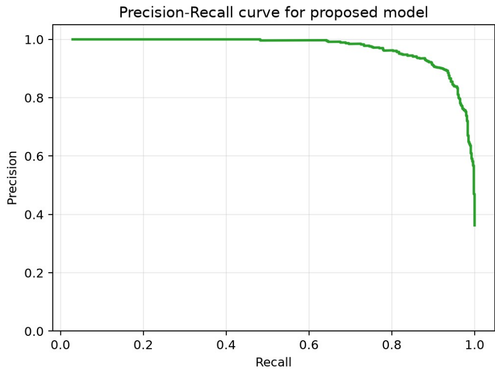
Рисунок 9 – Precision-Recall кривая proposed model
