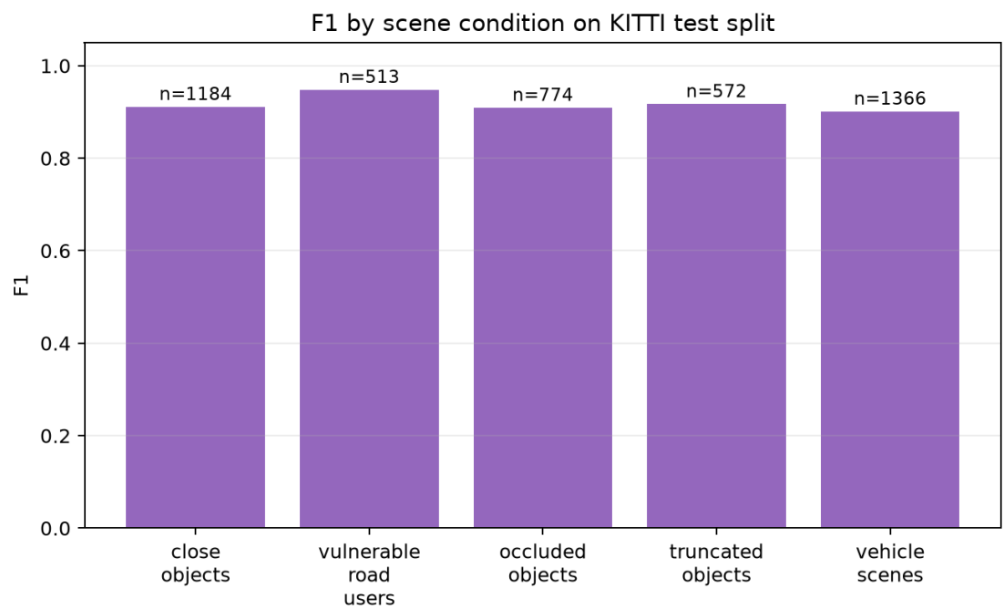
Рисунок 10 – F1 по группам сцен
