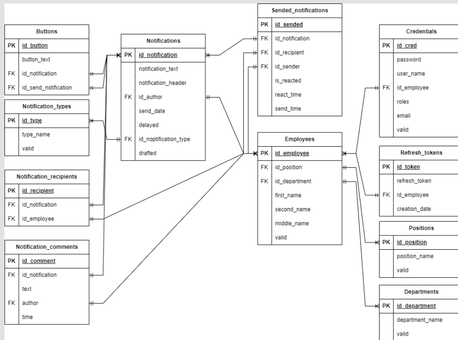
ER диаграмма базы данных
