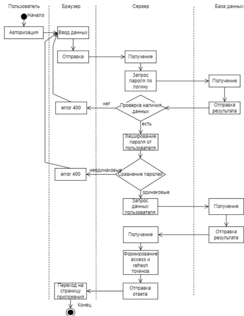
Рисунок 17 – Процесс авторизации
