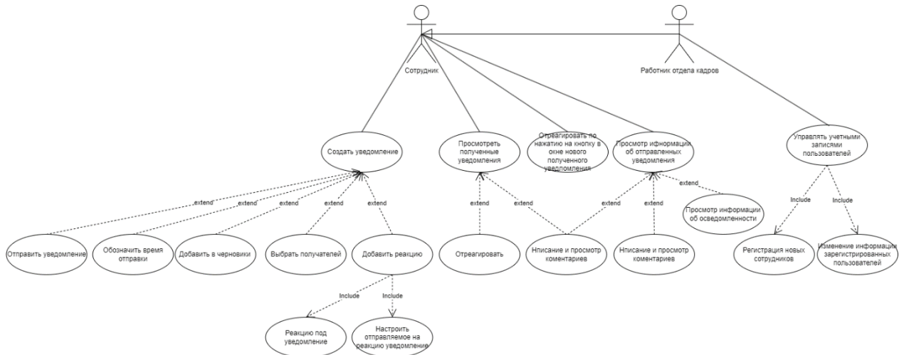
Рисунок 11 – Use-case диаграмма
