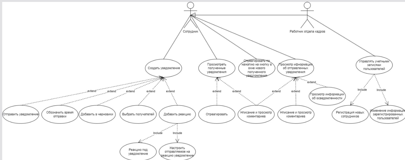
USE-CASE диаграмма
