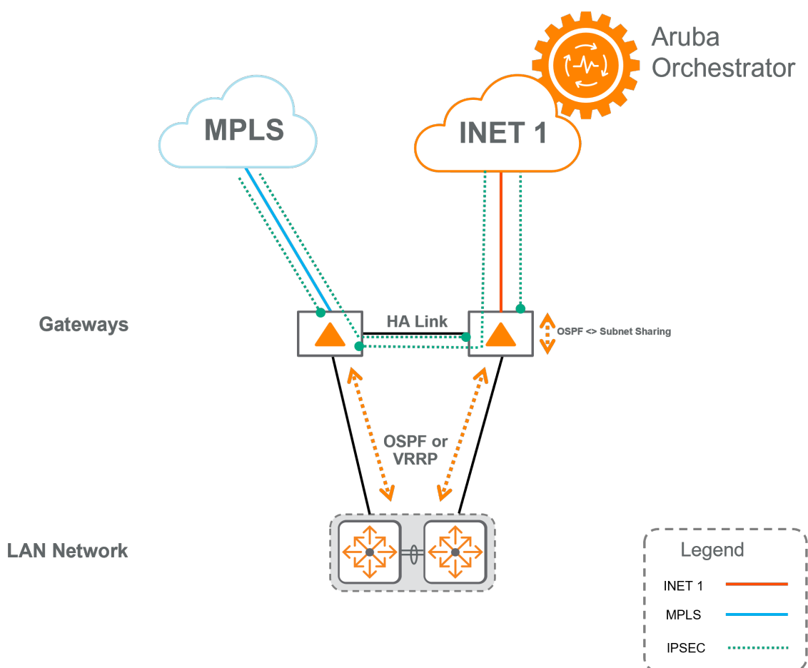
Figure 20: EC HA
