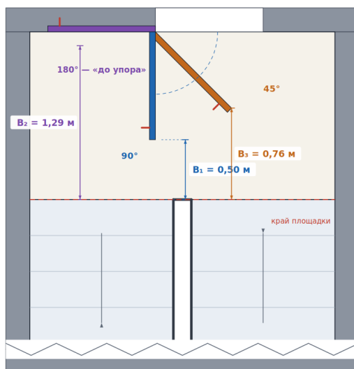
Рисунок 2. Что считать «максимально открытым положением»
