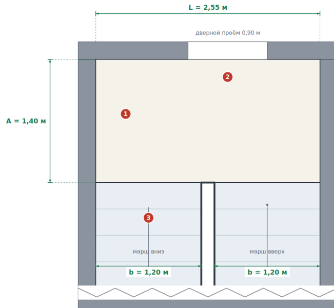
Рисунок 1. Исходная схема и обозначения размеров
