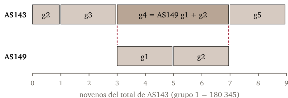
Figura 2. La distribución berlinese en novenos del total de AS143 (grupo 1). AS143 guarda un grupo de 4/9 (g4) que es igual, posición por posición, a las dos partes de 2/9 registradas por separado como grupos 1 y 2 de AS149.
