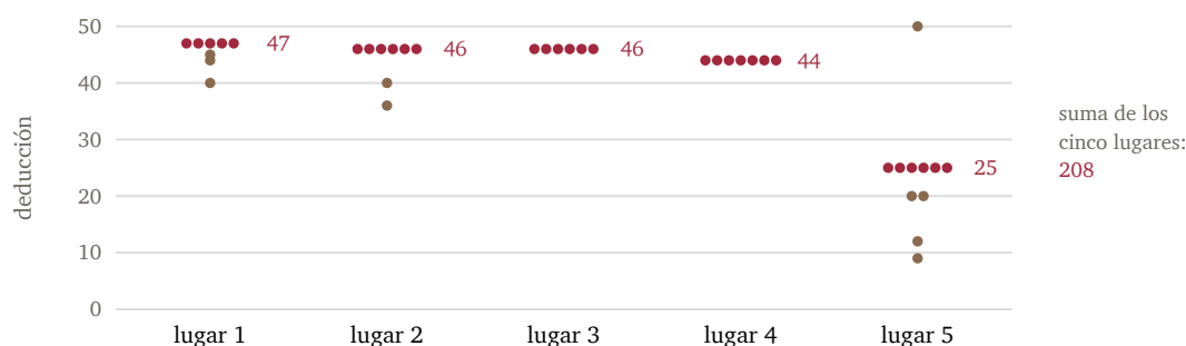
Figura 4. UR269: deducción de cada registro según su lugar en un bloque de cinco (bloques de al menos cuatro registros). En rojo, las deducciones iguales al valor más frecuente del lugar (33 de 43).
