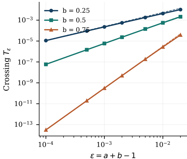
A. Power-law support edge
