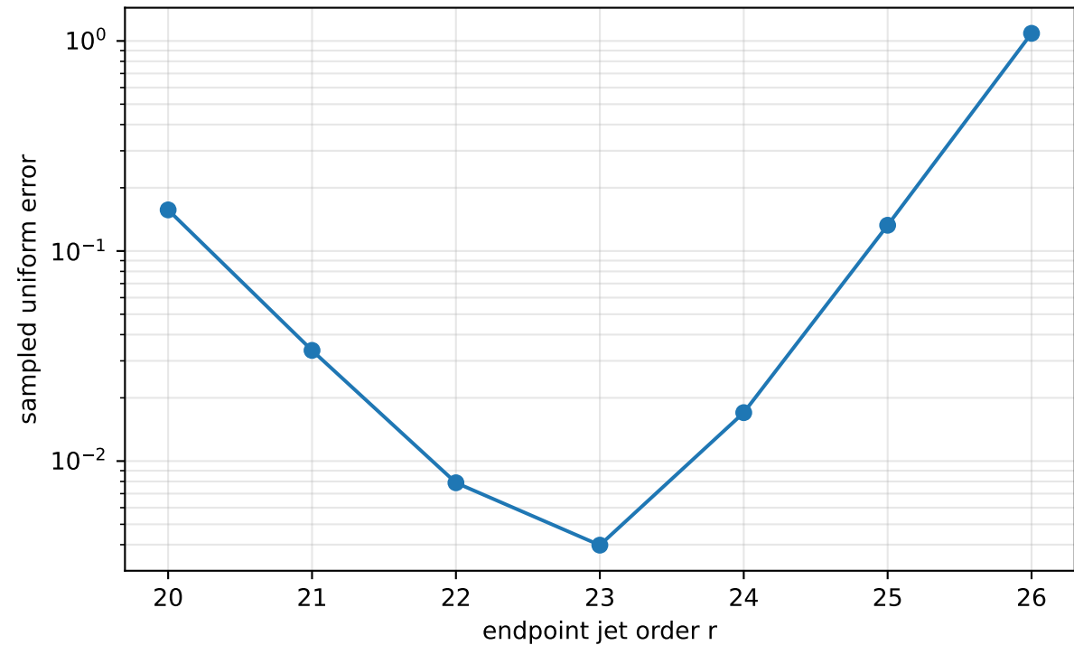
Endpoint-jet error scan, N=128
