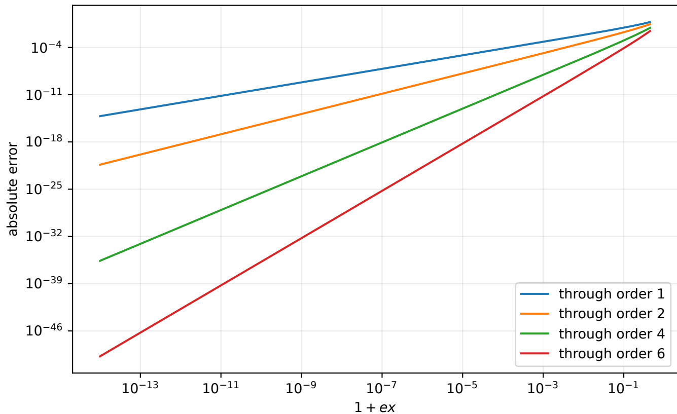
Puiseux approximation error for W_{-1}
