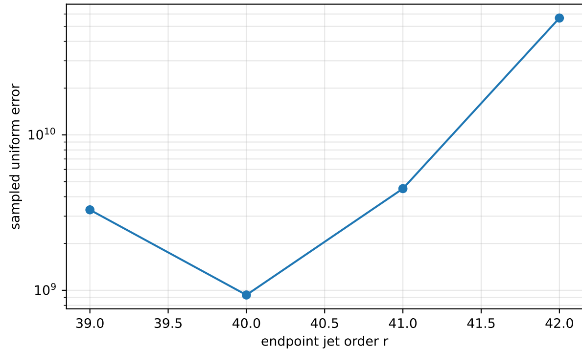
Endpoint-jet error scan, N=256
