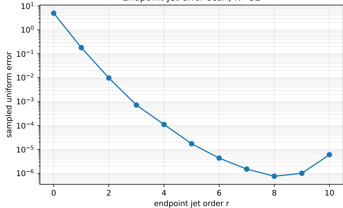
Endpoint-jet error scan, N=32
