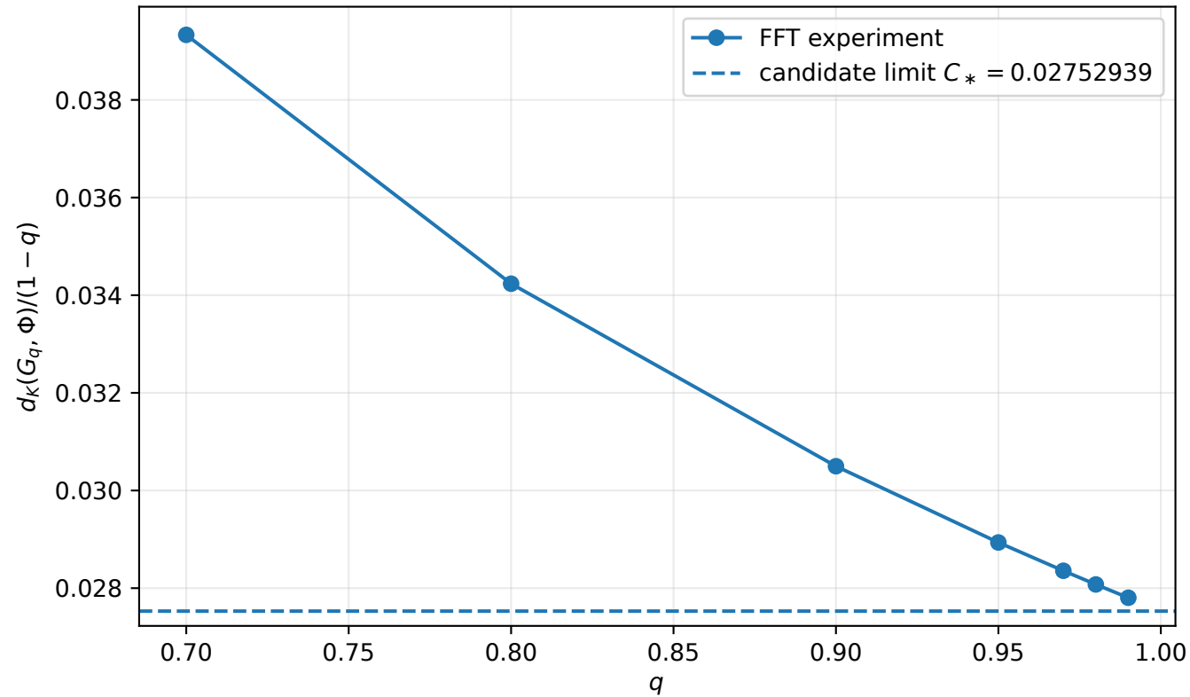
Kolmogorov-distance scaling
