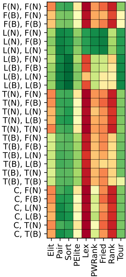
Population size 50
