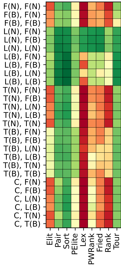
Population size 100
