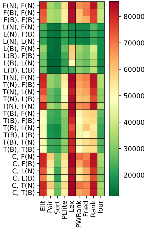
Population size 500
