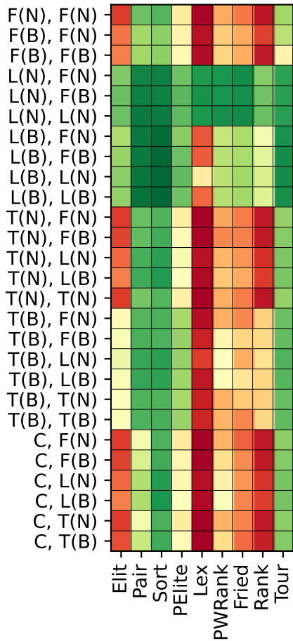
Population size 200
