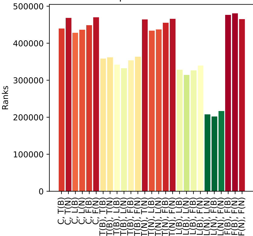
Population size 50
