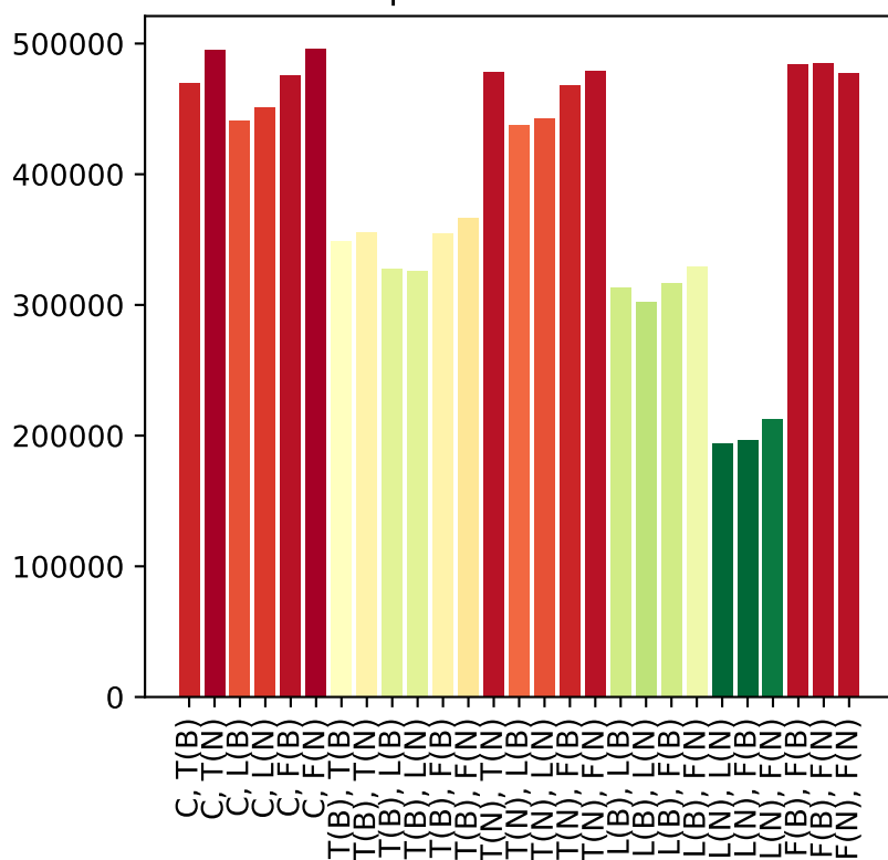
Population size 100
