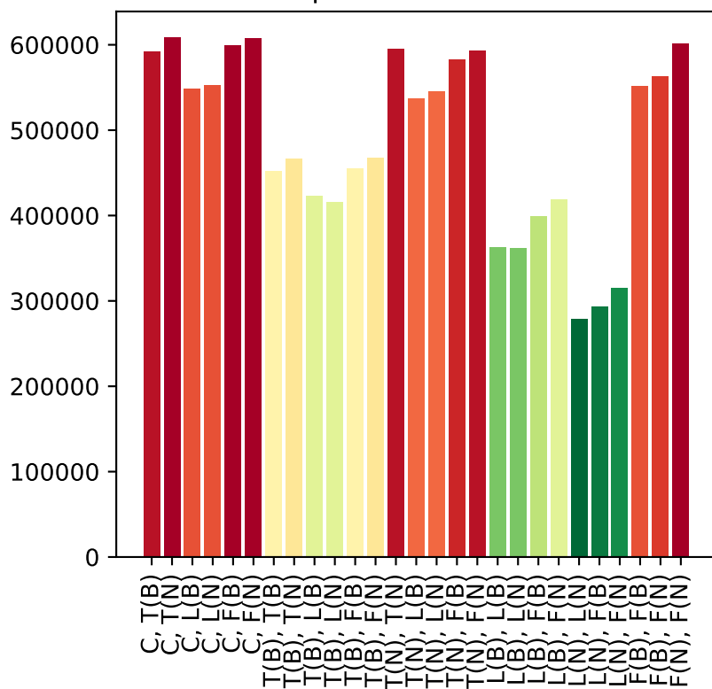
Population size 500
