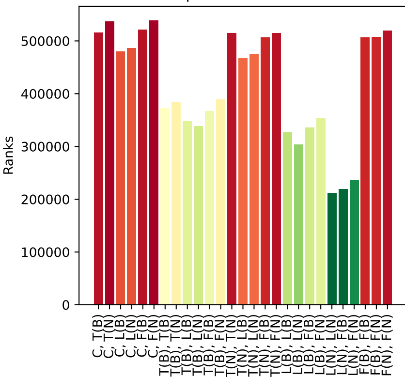
Population size 200
