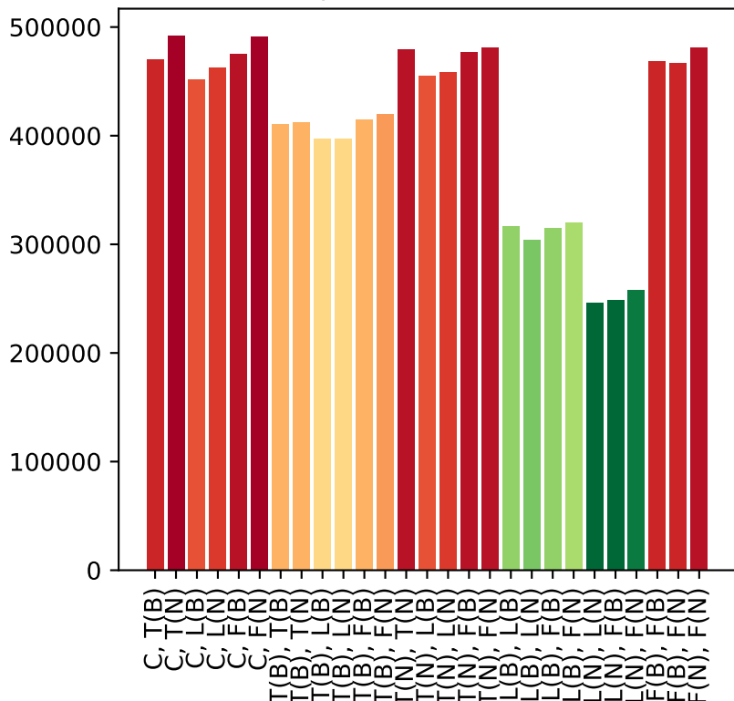
Population size 100
