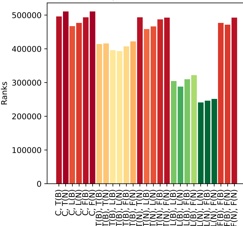
Population size 200
