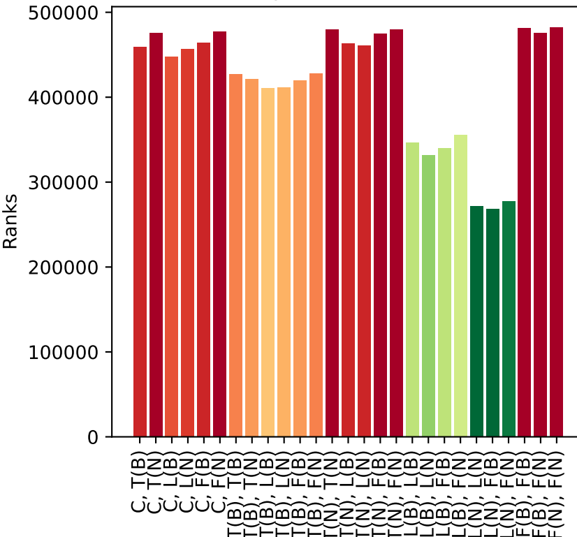
Population size 50
