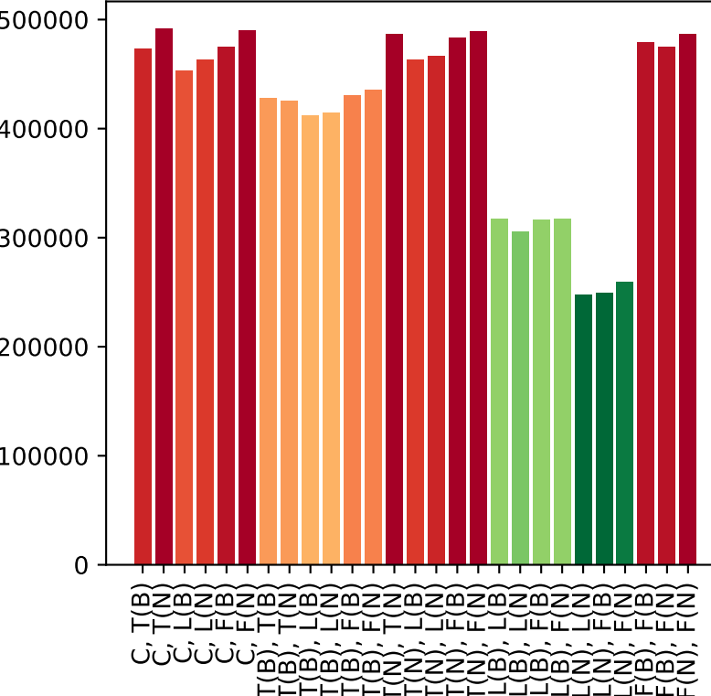
Population size 100
