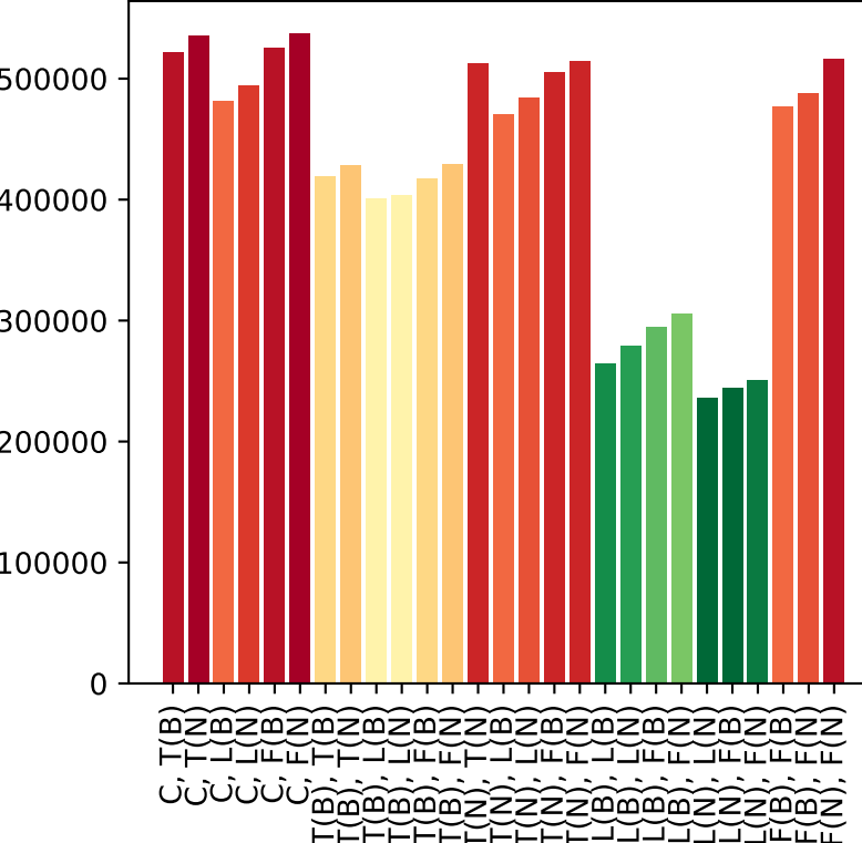
Population size 500
