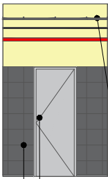
Плитка серая 300x300 Д-8 Проем 810x2100 (Замена) Потолок Армстронг водостойкий
