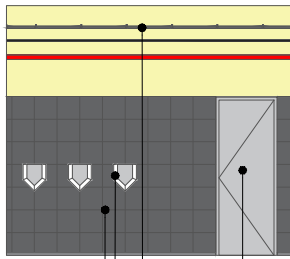
Плитка серая 300x300 111.6 Сушилка для рук Потолок Армстронг водостойкий Д-8 Проем 810x2100 (Замена)
