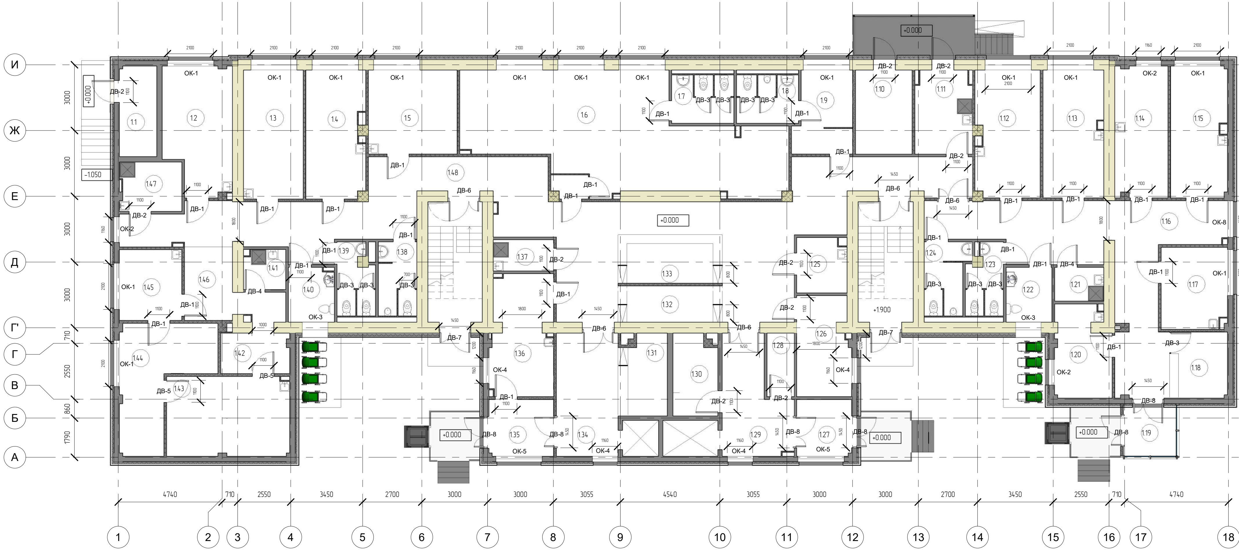
Схема расположения дверных и оконных проемов на плане +0.000 М 1:100
