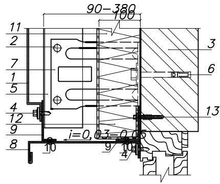
Узел Верх окна
