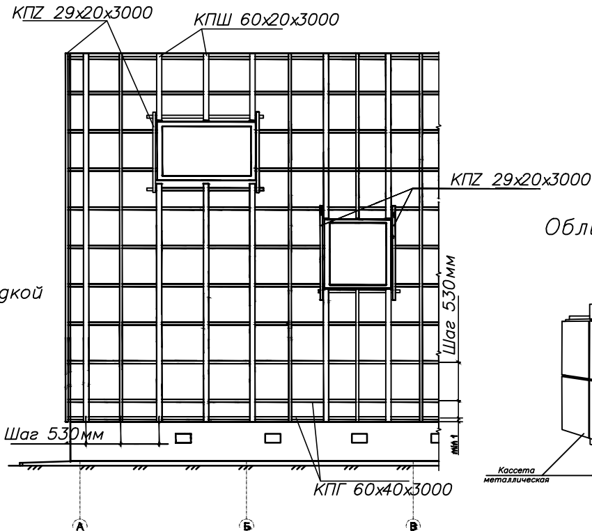
Система вентилируемого фасада Расположение горизонтальных и вертикальных направляющих при монтаже перекрестной подсистемы
