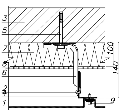
Узел Горизонтальный разрез
