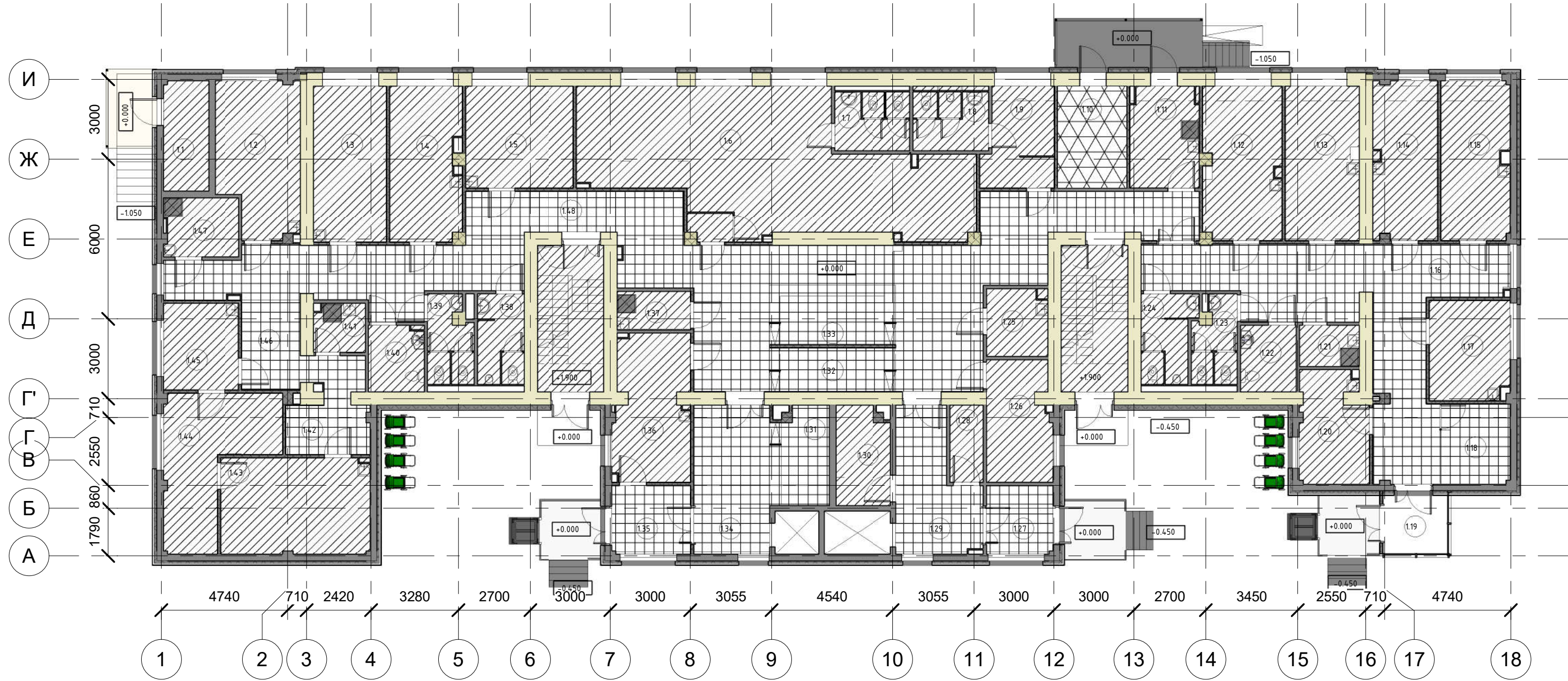
Схема монтажа потолков на 1 этаже
