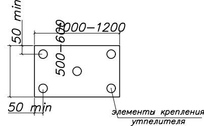
Система вентилируемого фасада Узел Крепление утеплителя рядовой плиты
