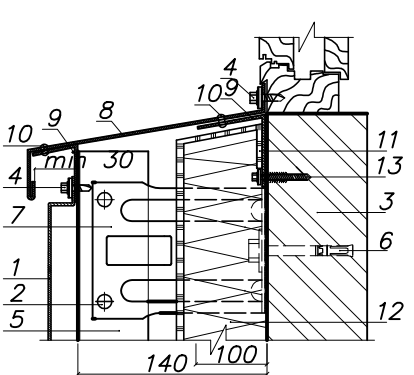
Узел Низ окна
