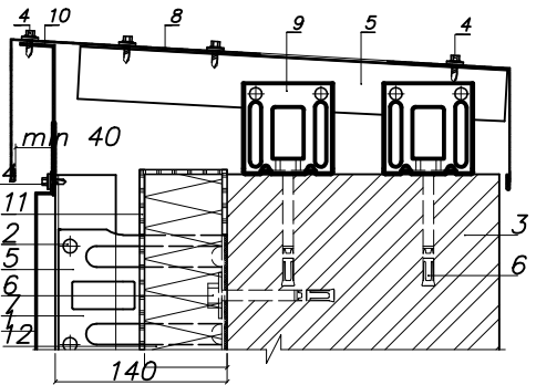
Система вентилируемого фасада Узел парапета
