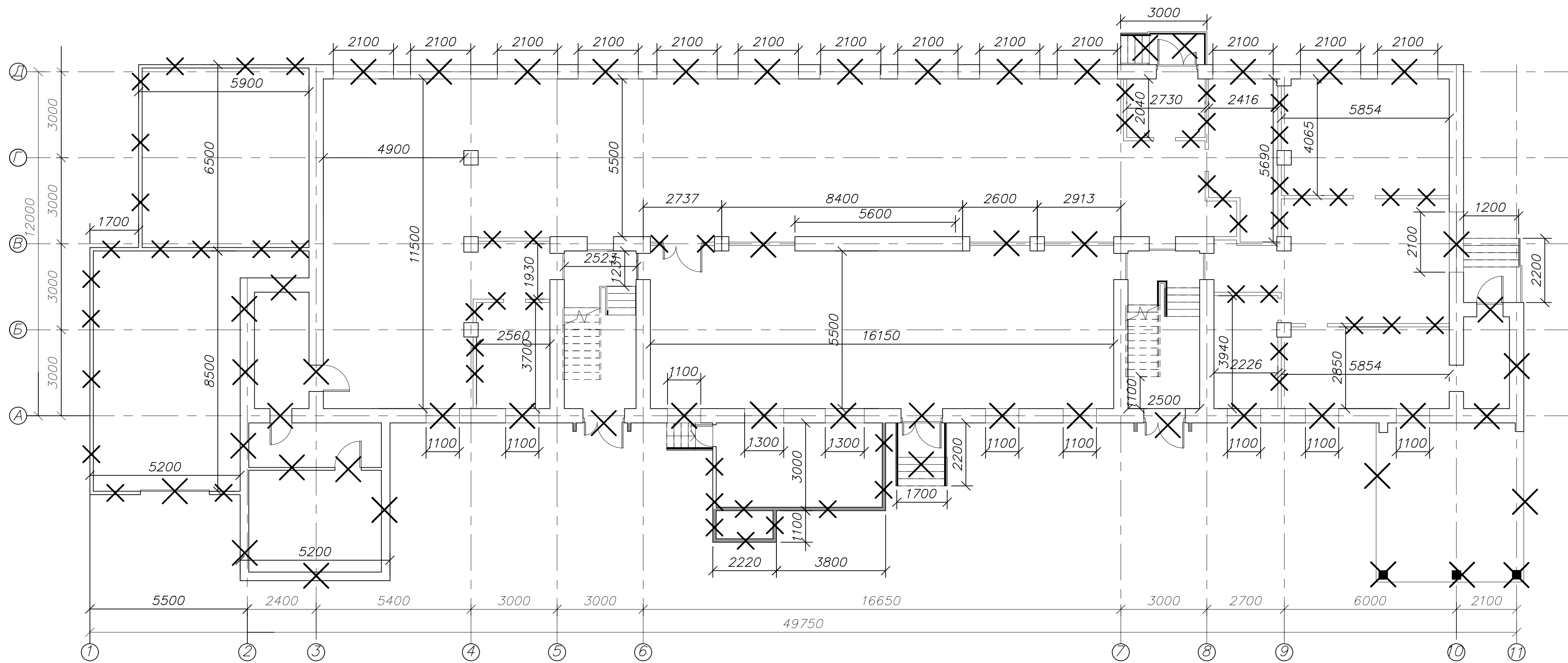
План 1-го этажа до реконструкции на отм. 0.000
