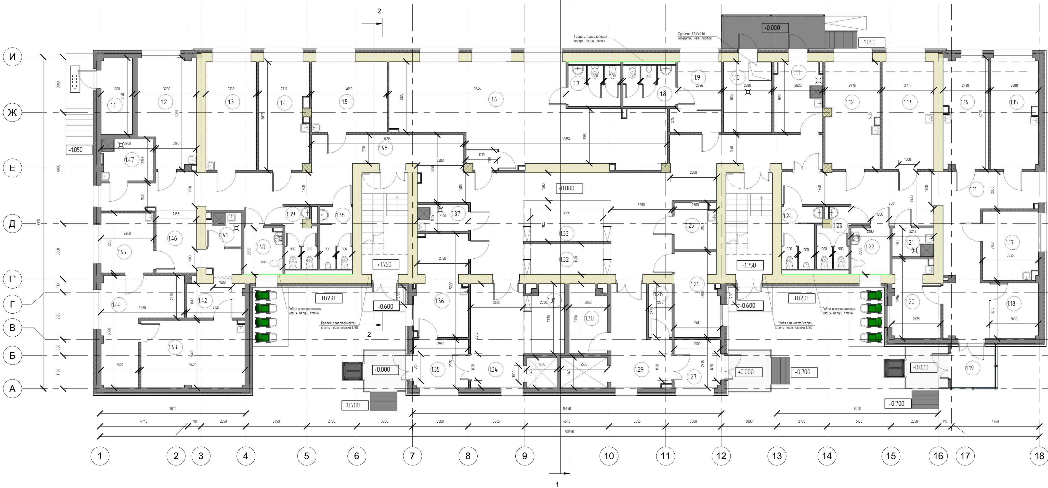
План на отметке +0.000 М 1:100
