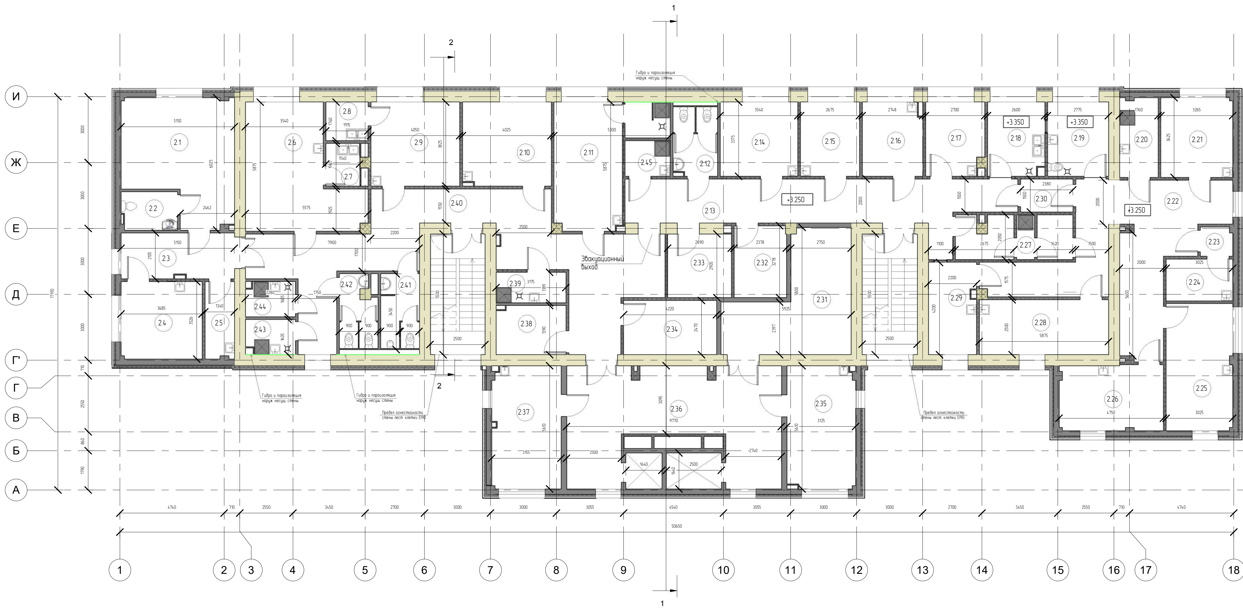
План на отметке +3.250 М 1:100
