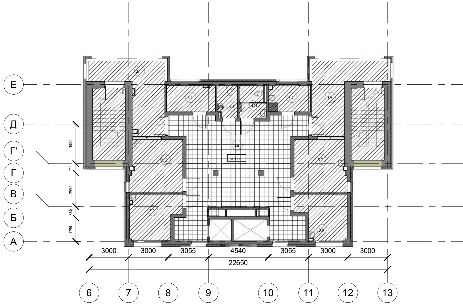
Схема монтажа потолков на 3 этаже
