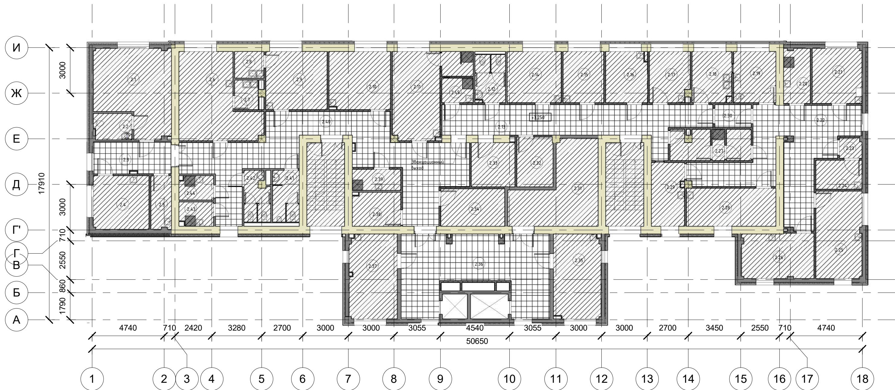
Схема монтажа потолков на 2 этаже
