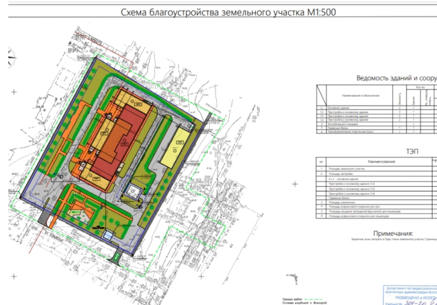
Схема благоустройства земельного участка
