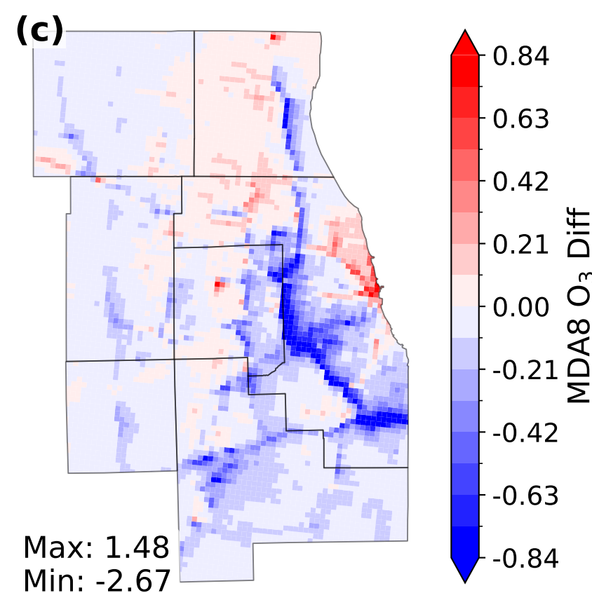
LOCUS Minus Default
